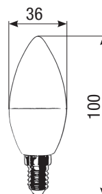
Abmessungen (mm) Dimensions (mm)
